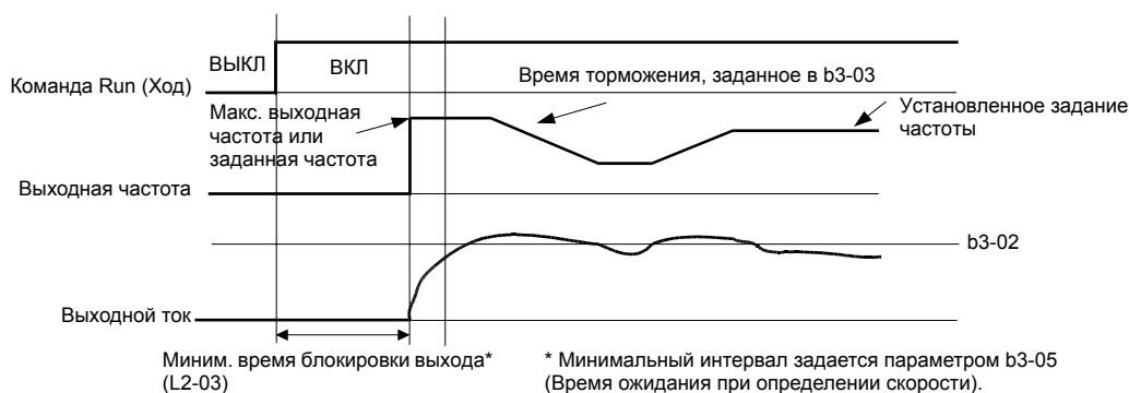
Рис. 6.35 Поиск скорости при пуске (определение тока)
