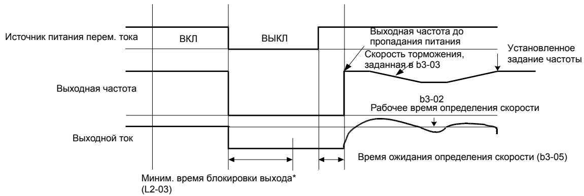
Рис. 6.37 Поиск скорости после блокировки выхода (определение тока; время пропадаания &gt; L2-03)
