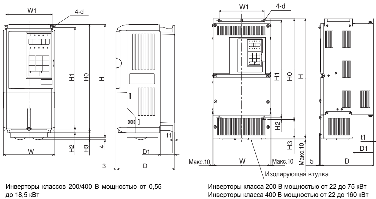
Рис. 1.10 Габаритные чертежи инверторов в исполнении NEMA 1 / IP20
