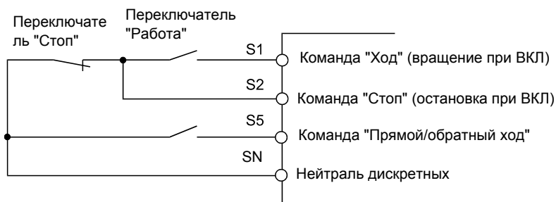
Рис. 6.12 Пример подключения при управлении по трем проводам
