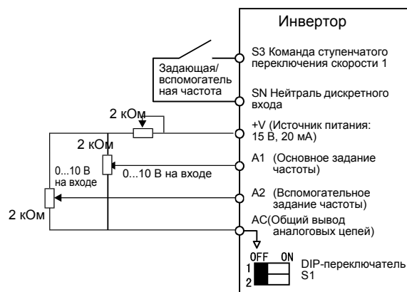
Рис. 6.7 Поддача основного/вспомогательного задания частоты
