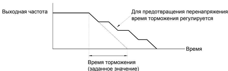
Рис. 6.22 Предотвращение опрокидывания ротора во время торможения
