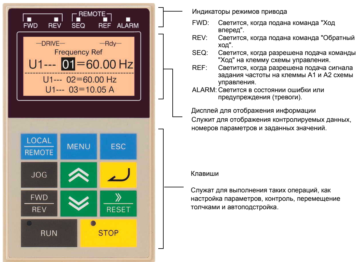
Рис. 3.2 Названия и функции элементов цифровой панели управления с ЖК-дисплеем
