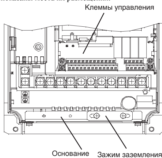
Рис. 2.16 Заземляющие зажимы инверторов IP54 мощностью от 7,5 до 18,5 кВт
