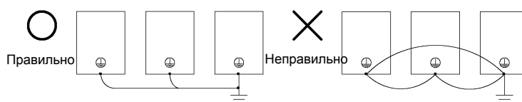
Рис. 2.9 Подключение заземления
