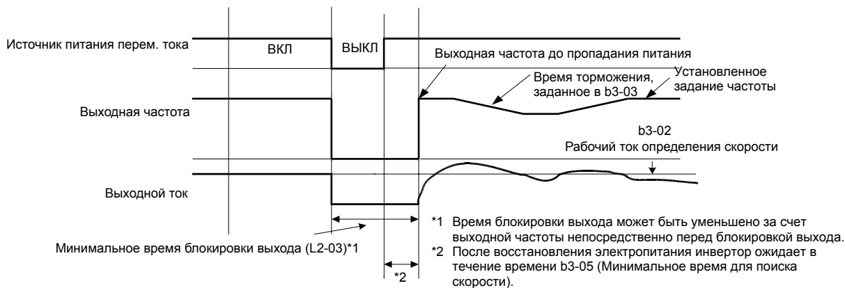
Рис. 6.36 Поиск скорости после блокировки выхода (определение тока; время пропадания < L2-03)
