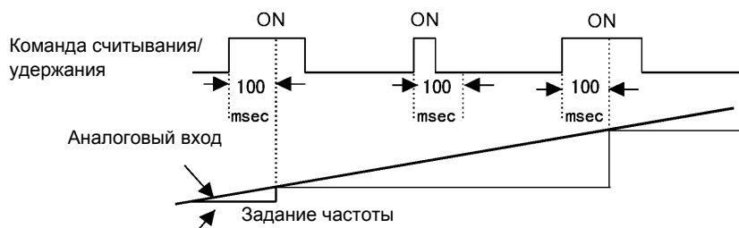
Рис. 6.46 Считывание/удержание аналоговой частоты
