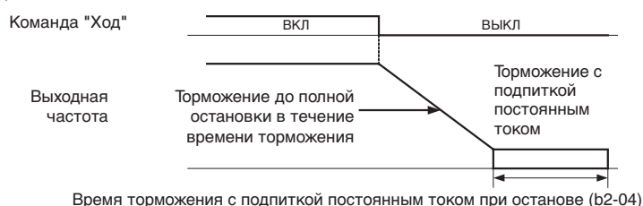
Рис. 6.14 Торможение до полной остановки
