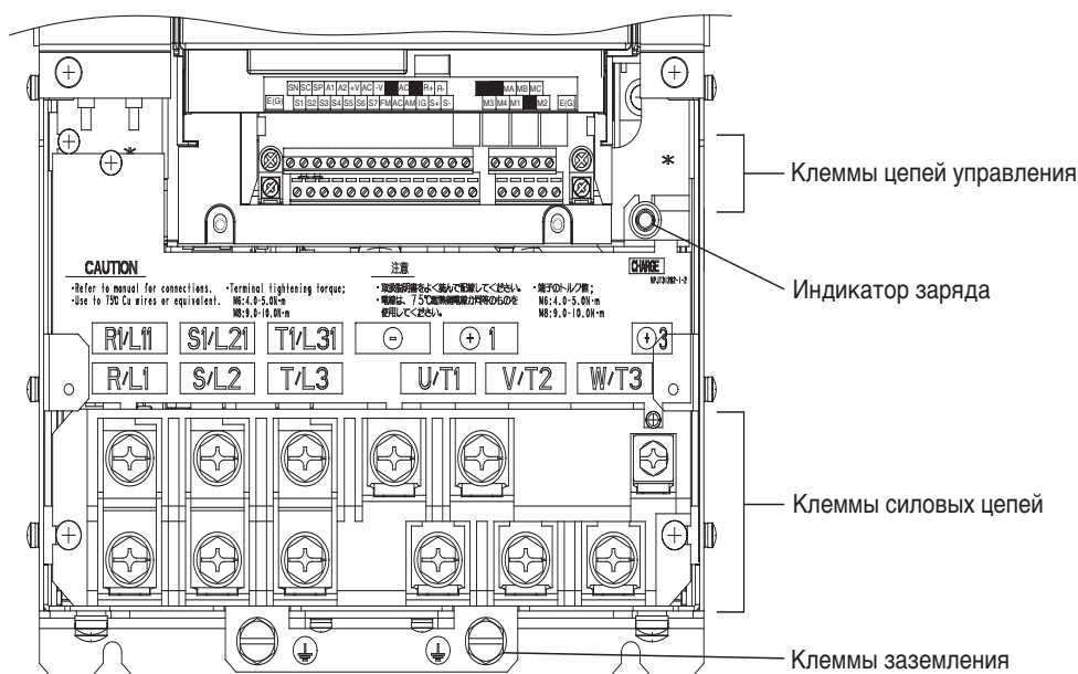
Рис. 2.4 Расположение клемм (инвертор класса 200 В/400 В, 22 кВт и больше)
