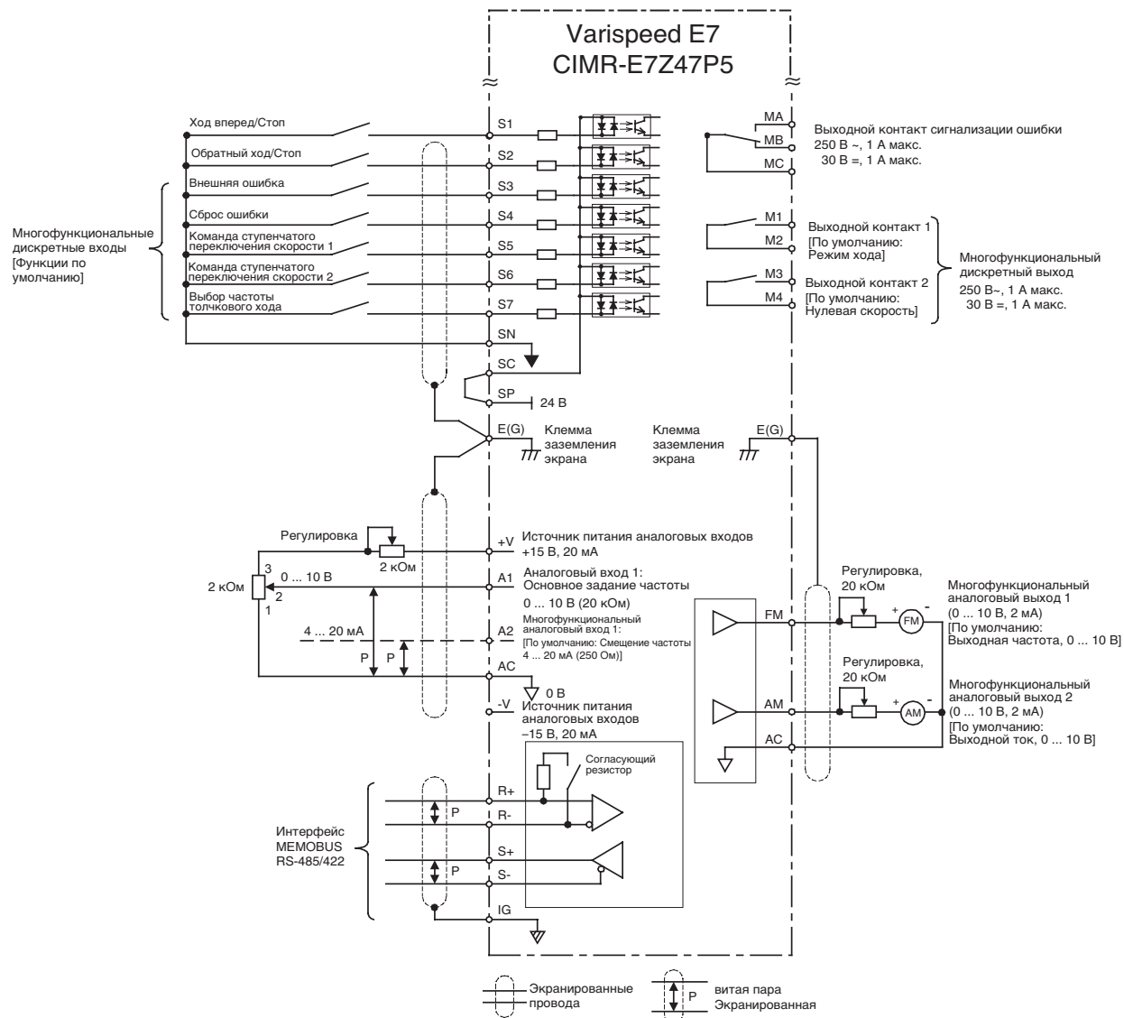
Рис. 2.21 Подключение клемм схемы управления
