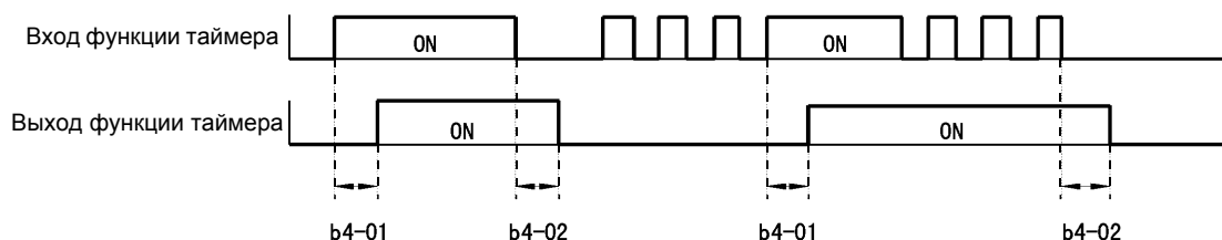
Рис. 6.55 Пример работы функции таймера
