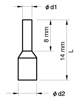
Рис. 2.14 Размер кабельного наконечника
