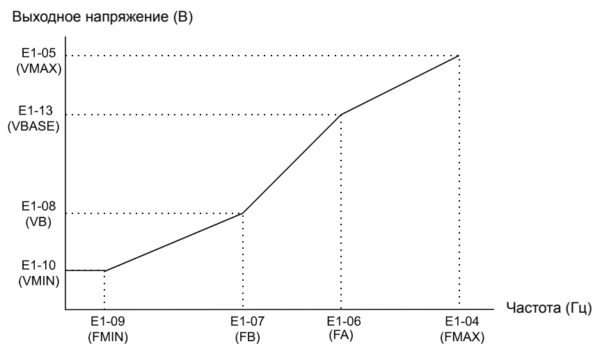
Рис. 6.62 V/f-характеристика пользователя
