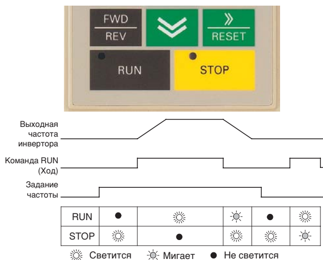
Рис. 3.3 Индикаторы RUN и STOP
