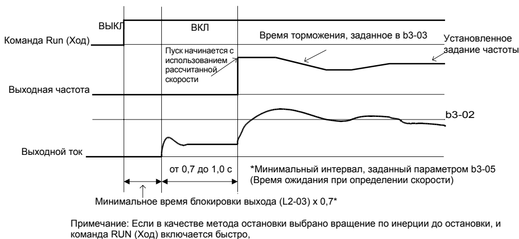
Рис. 6.32 Поиск скорости при пуске (с использованием рассчитанной скорости)
