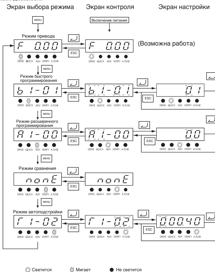
Рис. 3.4 Переключение режимов с помощью цифровой панели управления со светодиодным дисплеем
