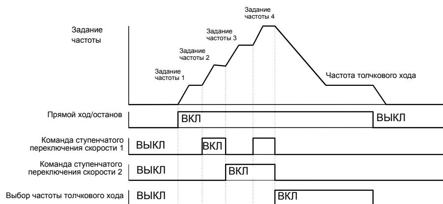
Рис. 6.10 Команды ступенчатого переключения скорости/выбора частоты толчкового хода. Временная диаграмма.
